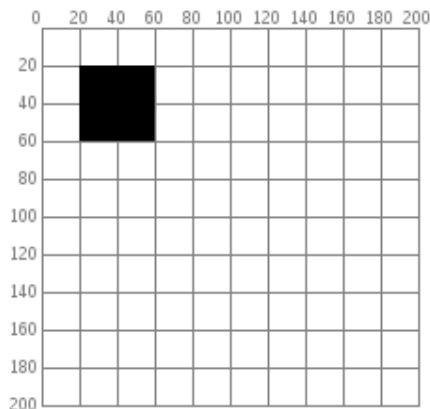
Gambar 3.1. Objek persegi sederhana
