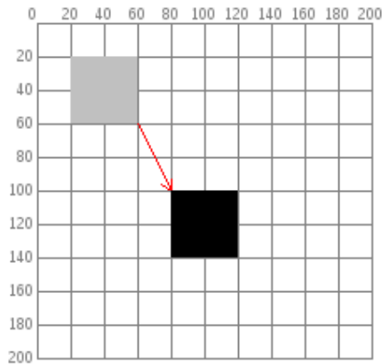
Gambar 3.2. Proses pemindahan objek dengan translasi
