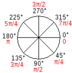
Gambar 3.4. Perbandingan sudut Radian dan Derajat
