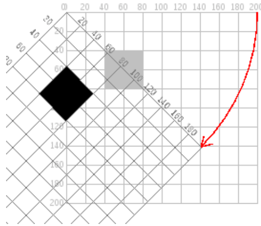
Gambar 3.5. Proses rotasi grid
